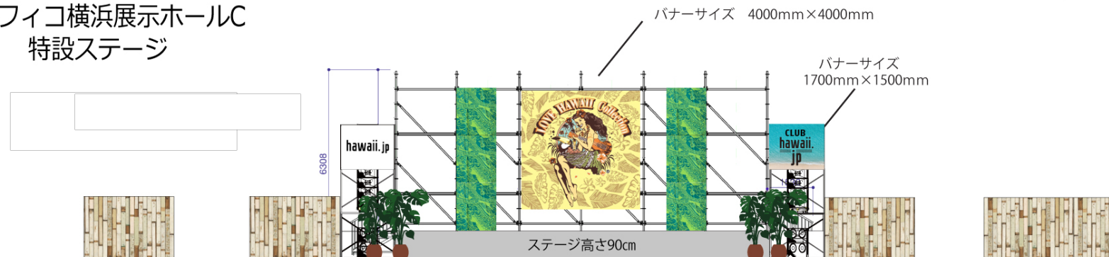
ステージ立面図
