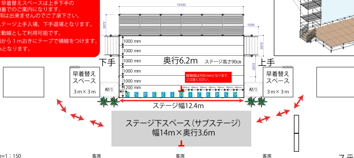
ステージ平面図
